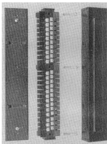
20 linjers kopplingsbox
