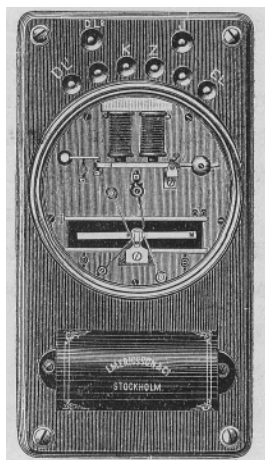
Signalöfverföringsapparat (F. O. Sjöströms patent) i förening med Bennets transformator.
