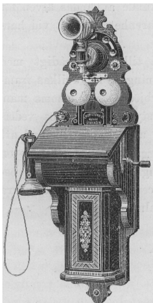
Väggapparat med kolkornsmikrofon. (L. M. Ericssons patent).
